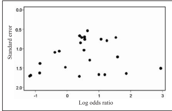
Şekil 1: Huni grafiği.
